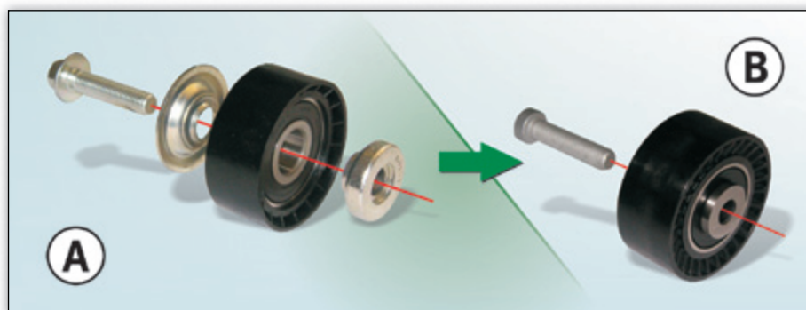
Polia de inversão 532 0433 10, versão anterior (A) e nova versão (B)
