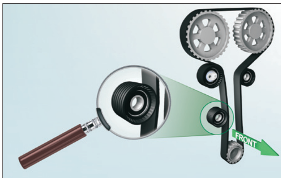
Fig. 1: Curso da correia e posições das polias no motor F4R
